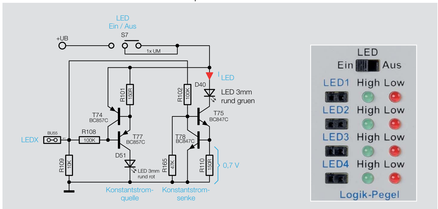
Bild 12: Ausschnitt aus dem Schaltungsteil „Logik-Pegel“ und dem zugehörigen Platinaufdruck
