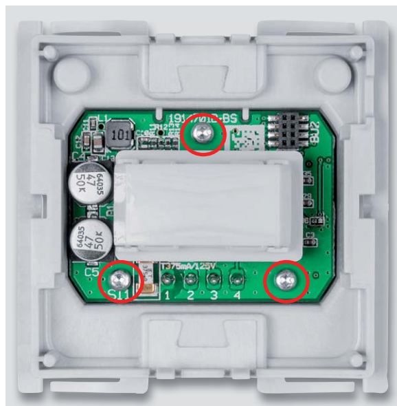
Bild 8: Die in das Gehäuseunterteil eingesetzte und verschraubte Basisplatine
