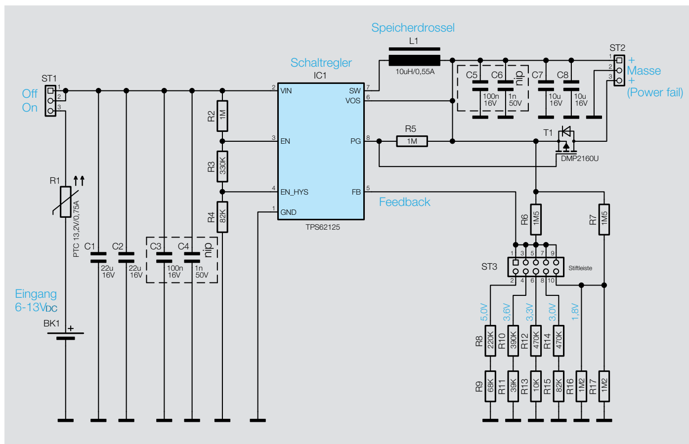
Bild 7: Schaltbild des BAP5
