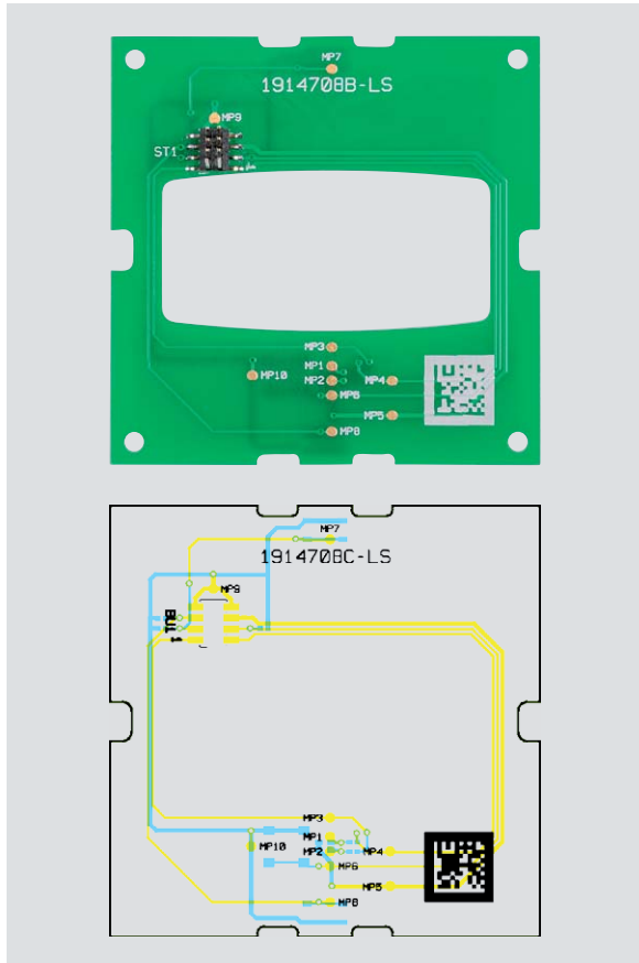
Bild 4b: Platinenfoto der bestückten Lötseite der Tasterplatine mit zugehörigem Bestückungsdruck
