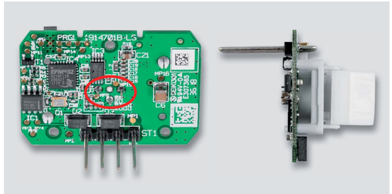
Bild 7: Das Einsetzen des Pyrosensor in die Platine – die Anschlüsse müssen genau in die zugehörigen Öffnungen fassen.
