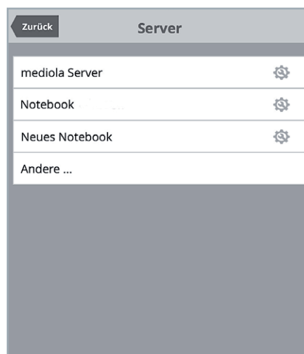
Bild 13: Serverliste
