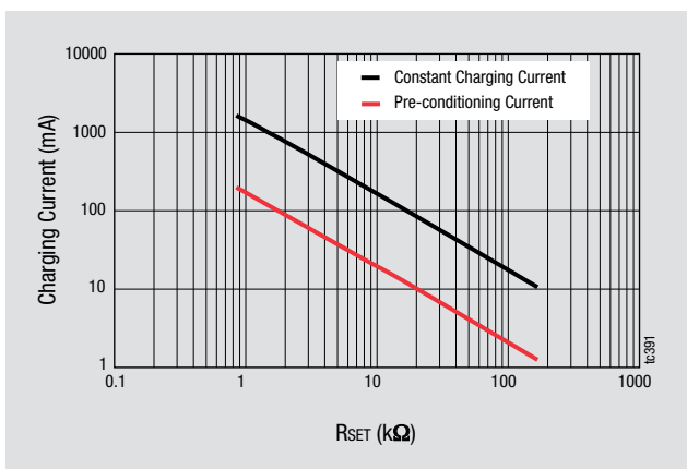
Bild 4: Abhängigkeit des Ladestroms und der Vorladung von der Widerstandsbeschlattung RSET
