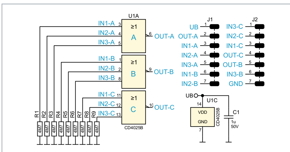
Bild 13: Schaltbild des Moduls CD4025
