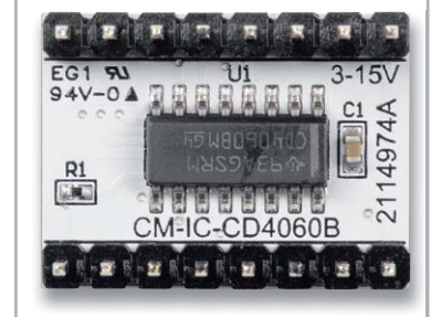
Bild 36: CD4060-Modul
