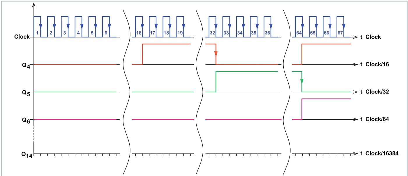
Bild 33: Signaldiagramm des CD4060
