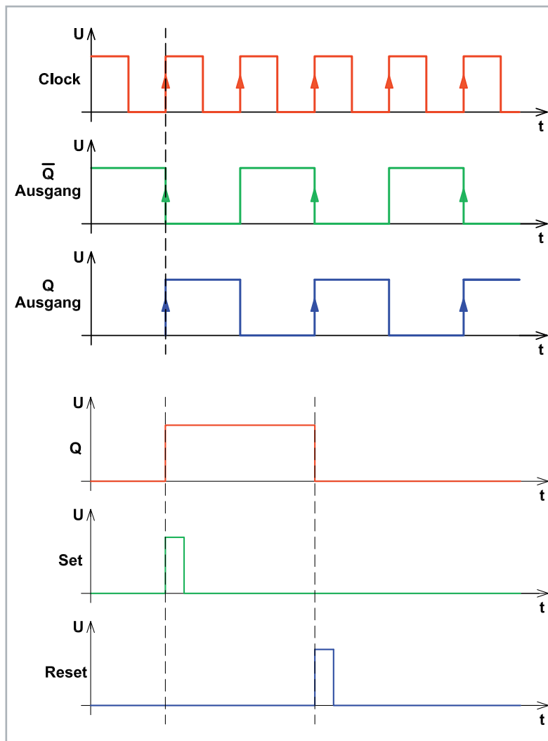
Bild 22: Die verschiedenen Modi des CD4013
