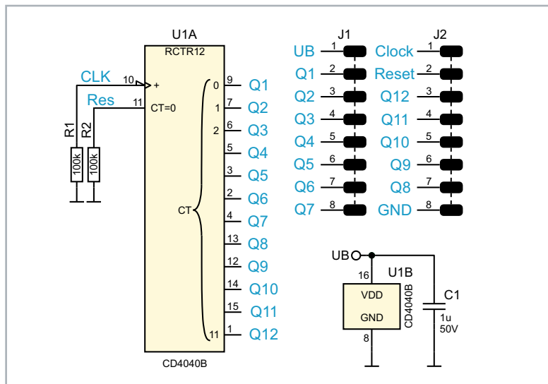
Bild 28: Schaltbild des CD4040
