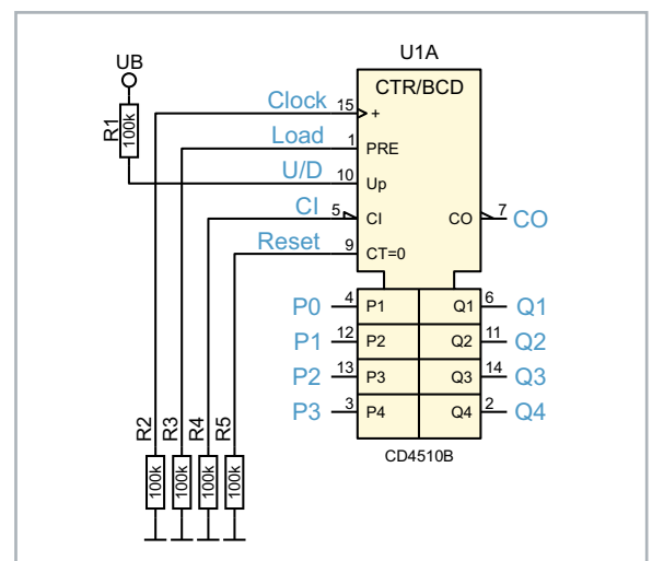
Bild 2: Schaltbild des CD4510
