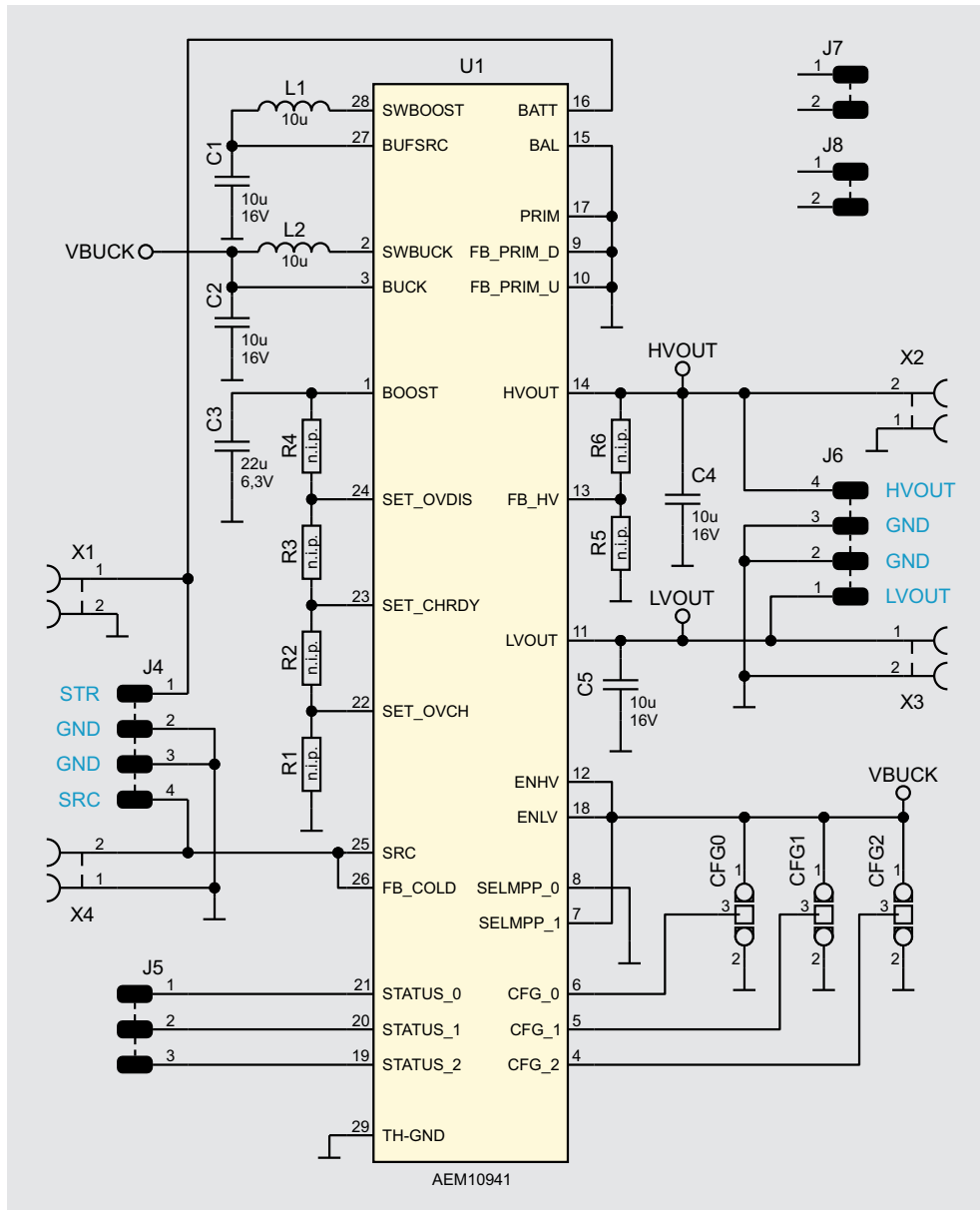
Bild 6: Schaltbild
