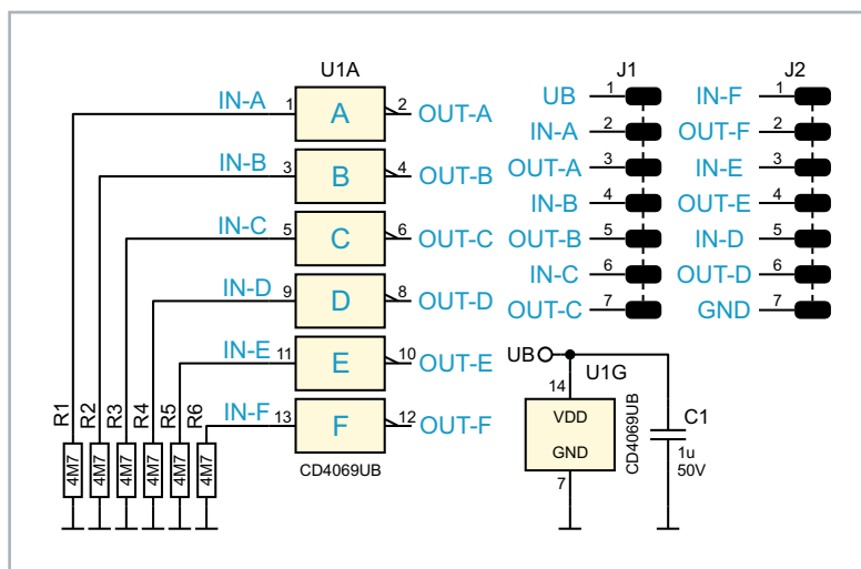
Bild 19: Schaltbild des Moduls CD4069
