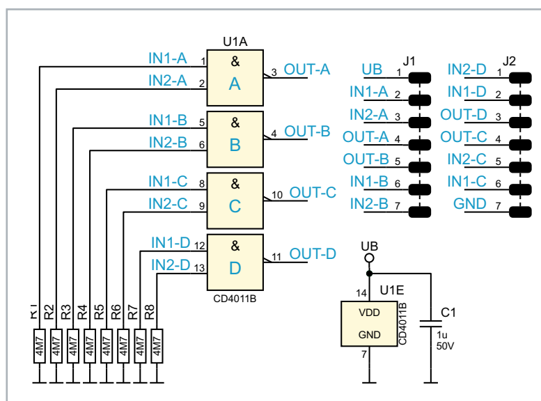
Bild 10: Schaltbild des Moduls CD4011
