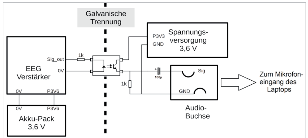
Bild 5: Anschluss des EEG-Verstärkers an den Mikrofon-Eingang eines Laptops
