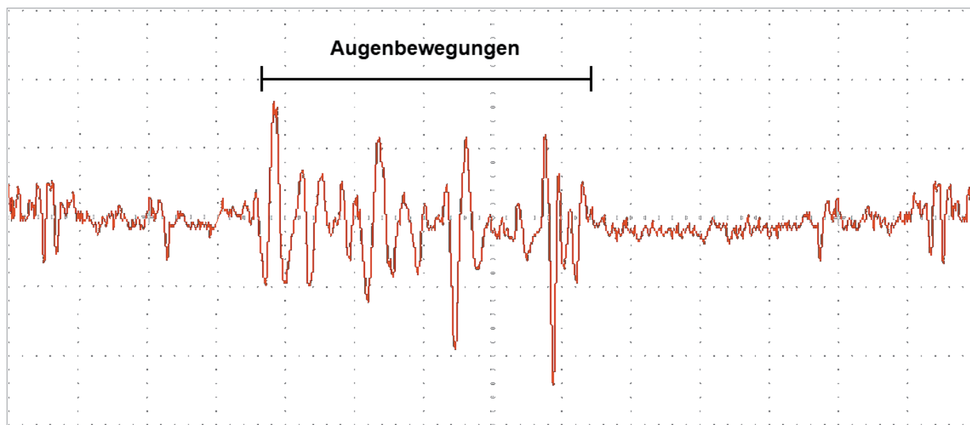
Bild 3: Augenartefakte
