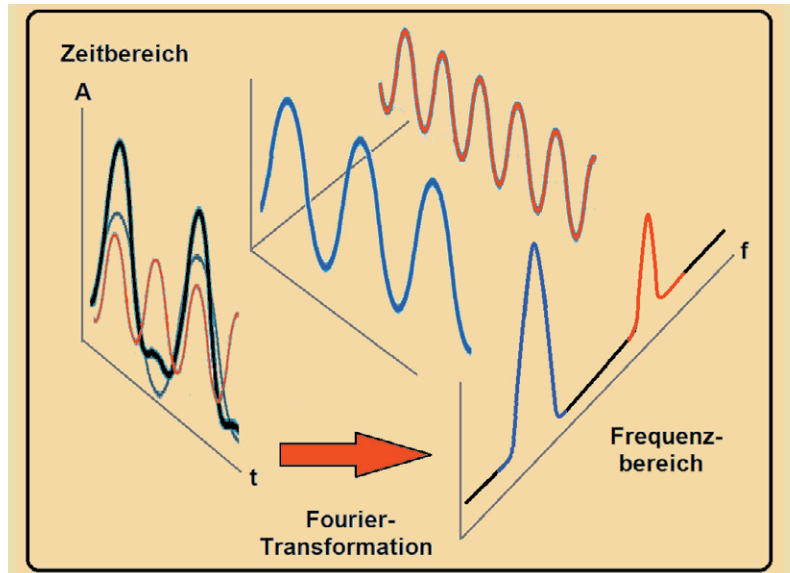
Bild 10: Prinzip der FFT
