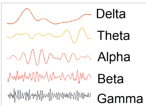
Bild 1: EEG-Signalformen
