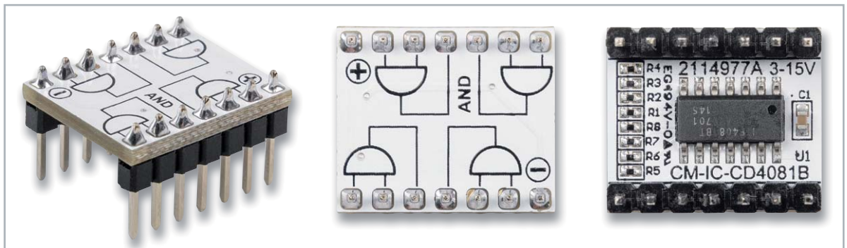
Bild 6: CD4081-Modul
