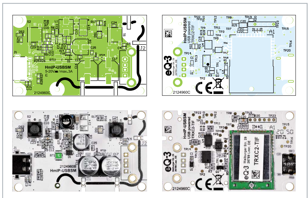
Bild 6: Platinenfotos und Bestückungspläne von der Bestückungsseite (links) und von der Lötseite (rechts)
