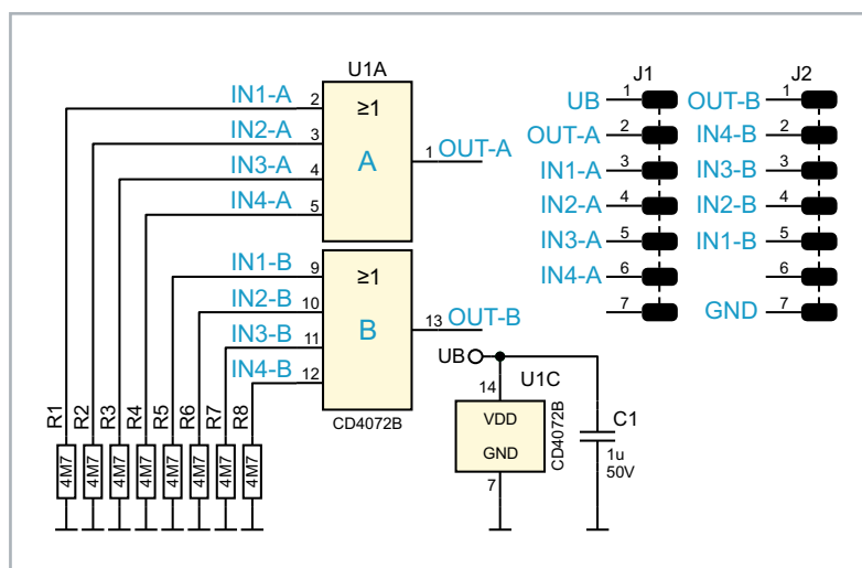
Bild 16: Schaltbild des Moduls CD4072
