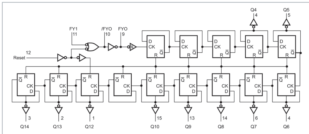
Bild 30: Blockschaltbild des CD4060 (Quelle: www.st.com)
