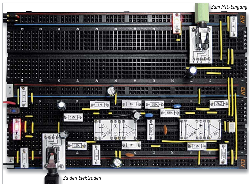
Bild 6: Aufbau zum EEG-Verstärker
