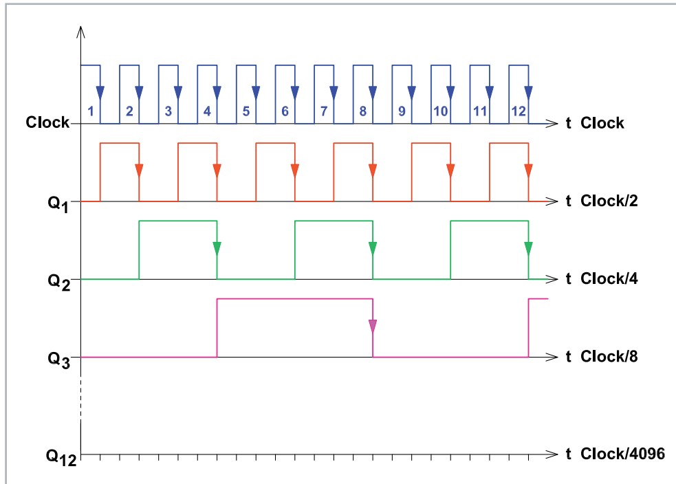
Bild 27: Signalverlauf des CD4040
