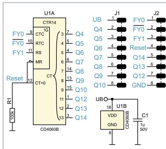
Bild 35: Schaltbild des CD4060
