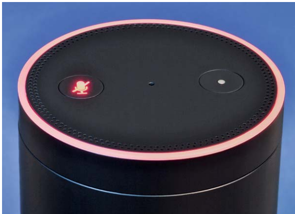
Bild 3: Deaktivierte Spracherkennung
