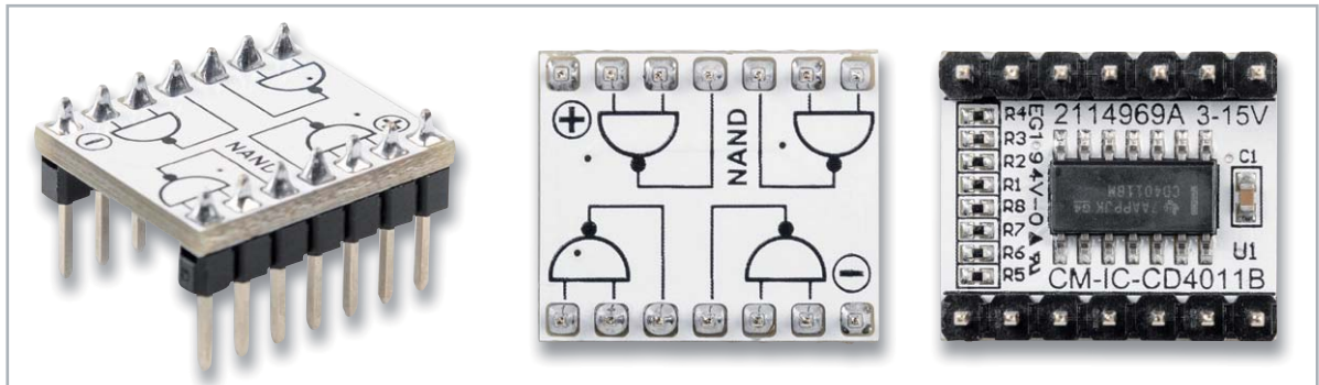
Bild 9: CD4011-Modul
