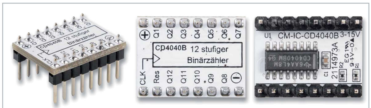
Bild 29: CD4040-Modul
