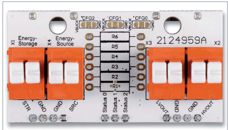
Bild 10: Bestückung der Federkraftklemmen
