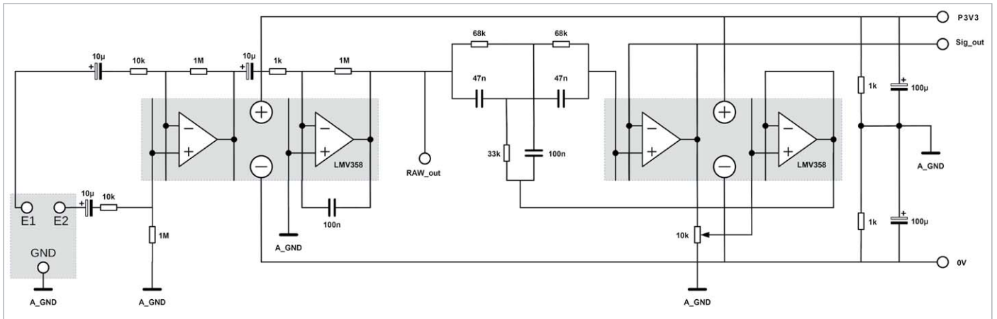
Bild 4: EEG-Vorverstärker
