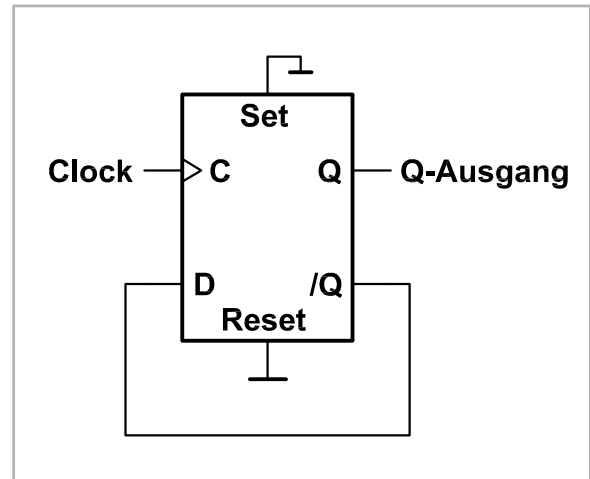
Bild 21: So wird aus einem D-Flip-Flop ein T-Flip-Flop.
