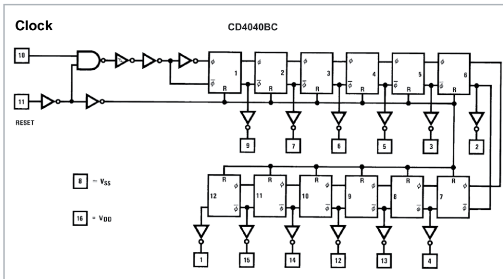
Bild 25: Blockschaltbild des CD4040
