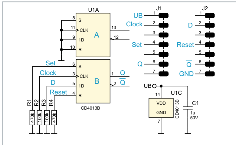
Bild 20: Schaltbild des Moduls CD4013
