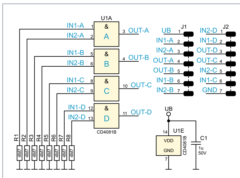
Bild 7: Schaltbild des Moduls CD4081
