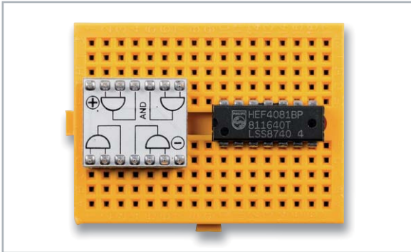
Bild 3: Einige PAD6-Module sind Pin-kompatibel mit DIP-Bausteinen.
