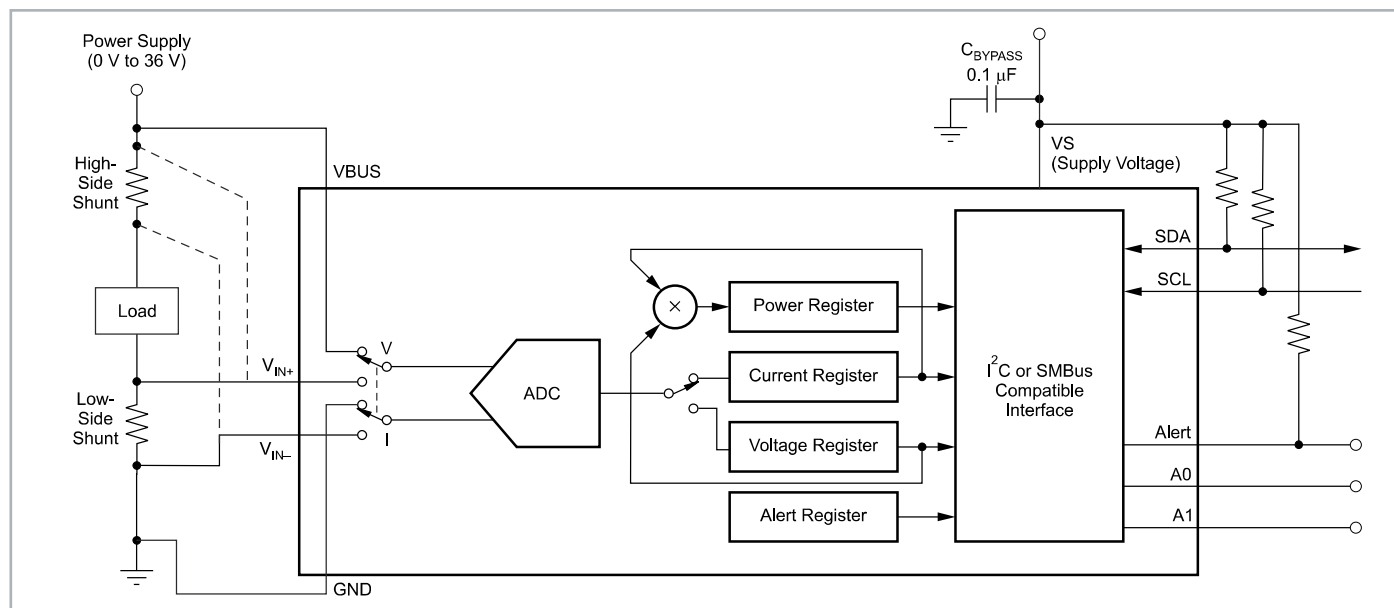
Bild 3: Anwendungsbeispiel INA226 (Quelle: Datenblatt Texas Instruments INA226)
