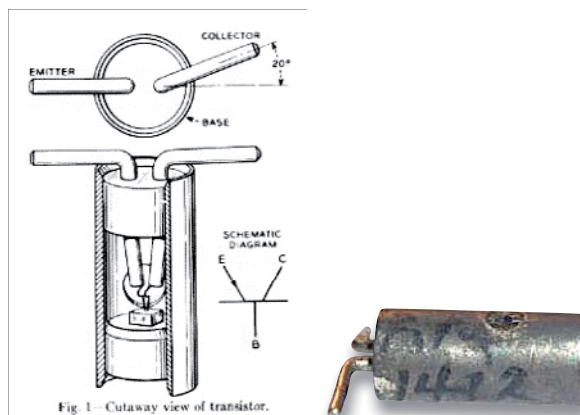
Bild 8: Der berühmte „Type A“-Transistor von Bell im Metallgehäuse war der erste in Serie gefertigte Transistor. Bilder: Copyright 2001-2017 by Jack Ward, transistormuseum.com
