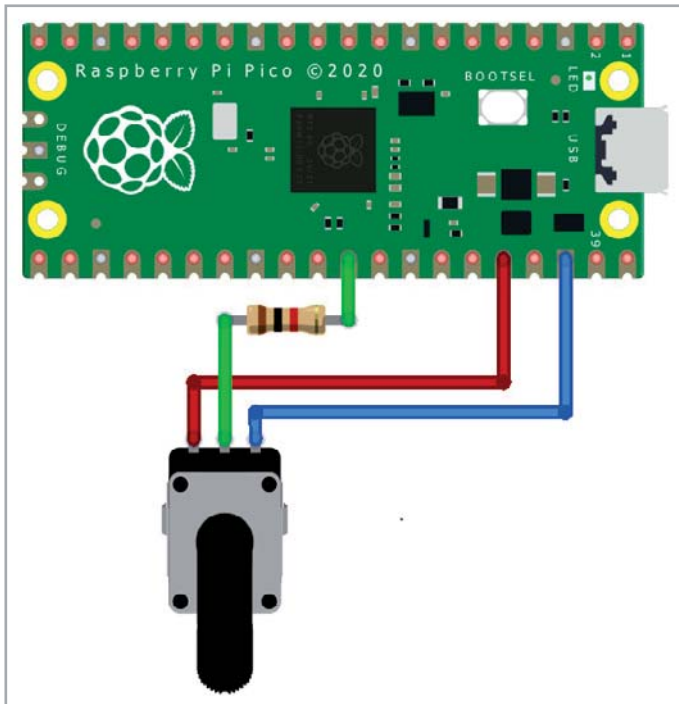
Bild 4: Potentiometer am Pico
