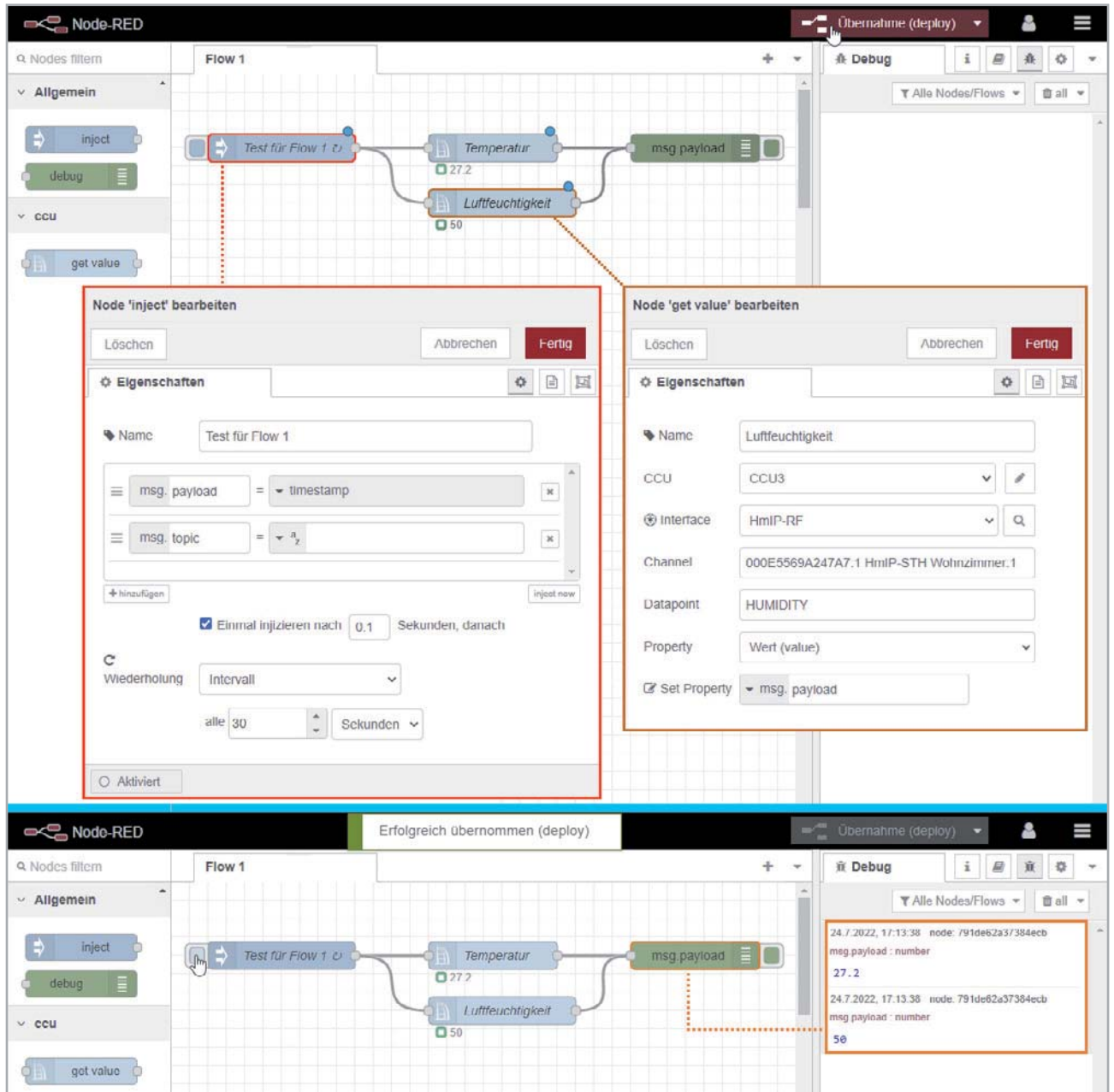
Bild 12: Ein erster Flow mit dem Luftfeuchtigkeitssensor HmIP-STH
