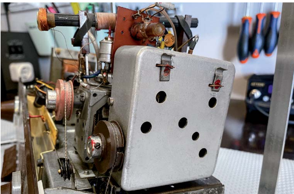
Bild 2: Das UKW-Frontend ist abgeschirmt, um die Stabilität zu gewährleisten und die Rauschaufnahme zu reduzieren.
