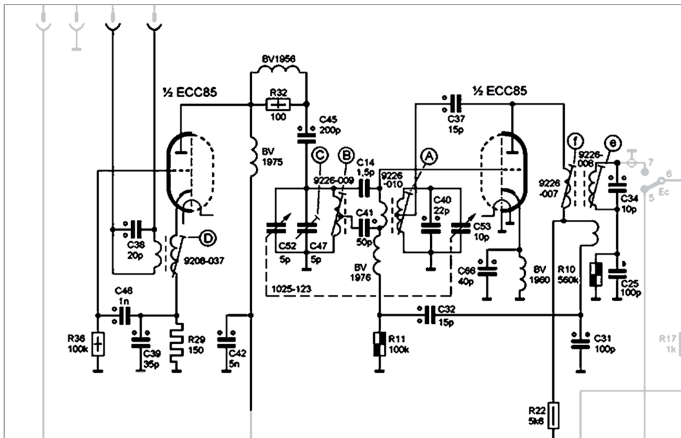
Bild 3: Schaltplan des UKW-Frontends
