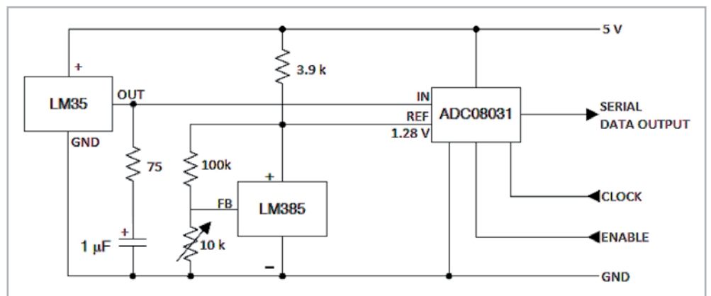
Bild 10: Der LM35 mit einem nachgeschalteten ADC, der ein serielles Digitalsignal ausgibt. Grafik: Texas Instruments
