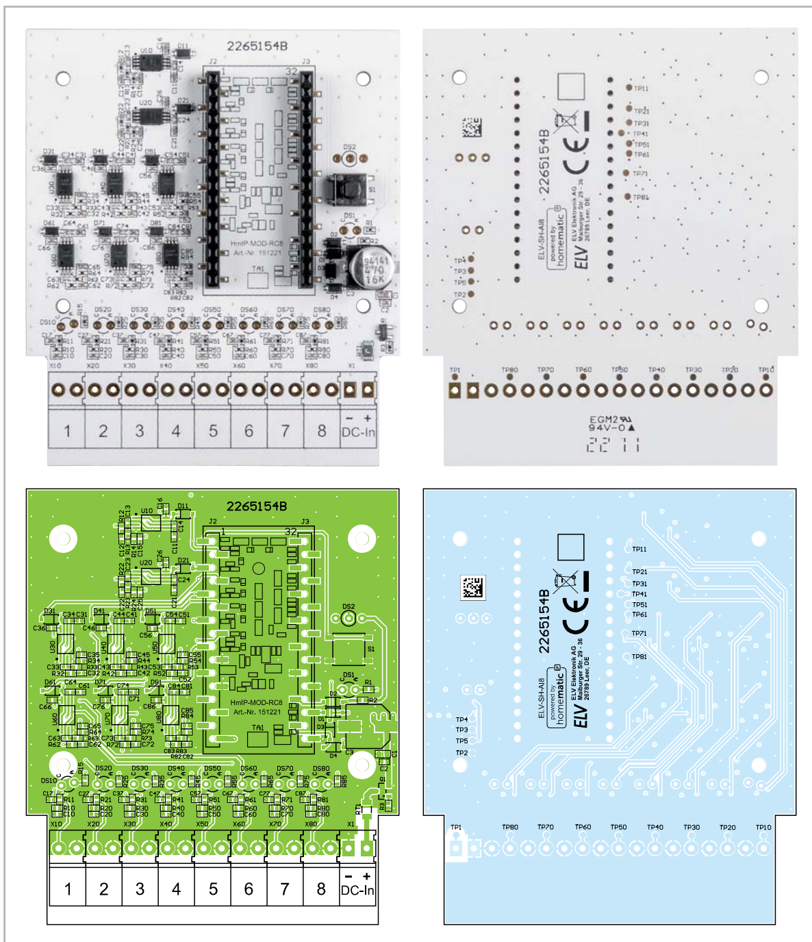
Bild 8: Platinenfotos und Bestückungsdrucke des Bausatzes ELV-SH-AI8
