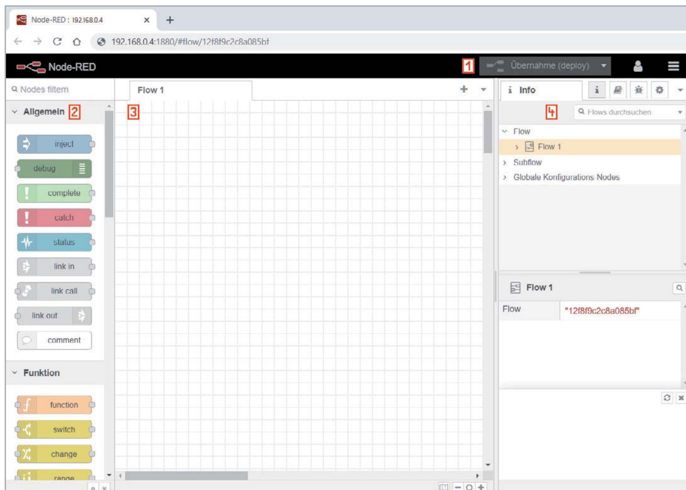
Bild 8: Node-RED-Startseite
