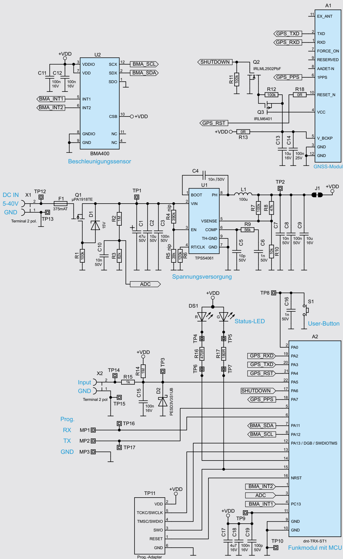
Bild 2: Das Schaltbild des ELV-LW-GPS1
