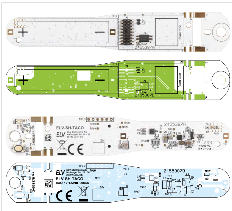
Bild 4: Platinenfotos und Bestückungsdrucke des ELV-SH-TACO
