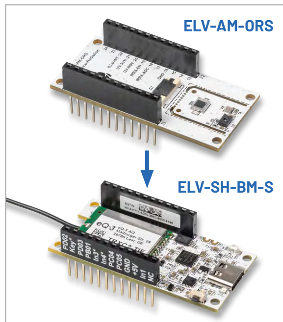
Bild 6: So wird das Applikationsmodul ELV-AM-ORS auf die Base - hier die ELV-SH-BM-S - aufgesetzt.
