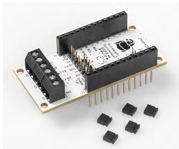
Bild 2: Lieferungsumfang des Interface ELV-AM-INT1
