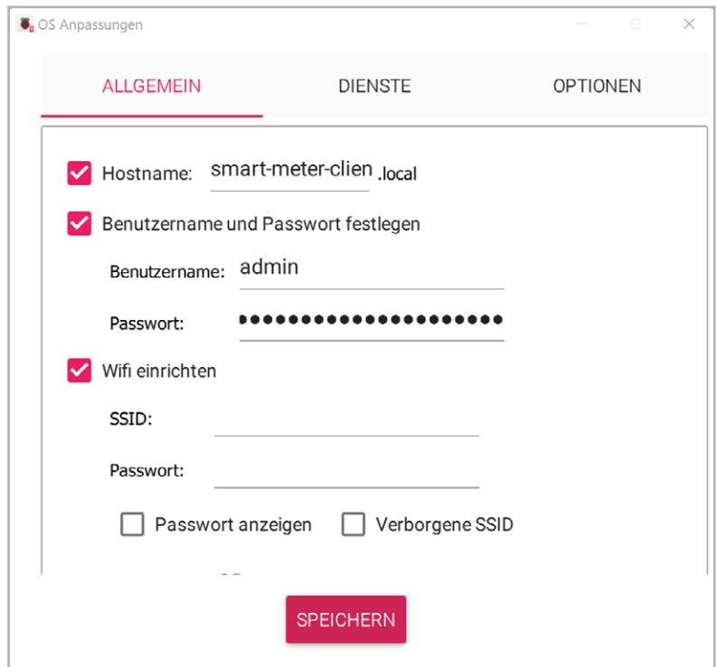
Bild 3: OS-Anpassungen
